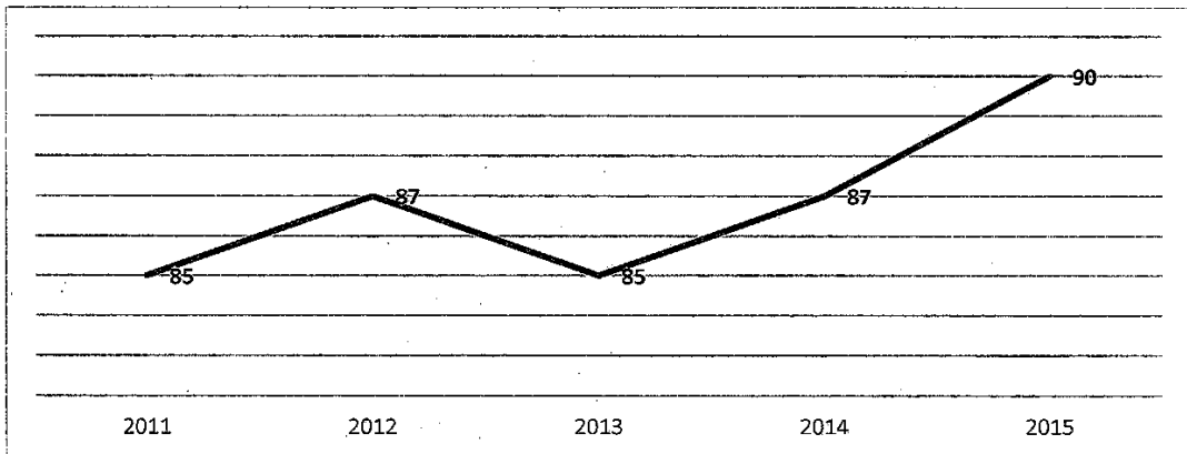
Figura 4.15 Índice Metropolitano de la Calidad del Aire (IMECA) promedio, 2011-2015
